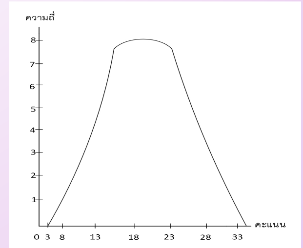
เส้นโค้งความถี่ (Frequency Curve)
