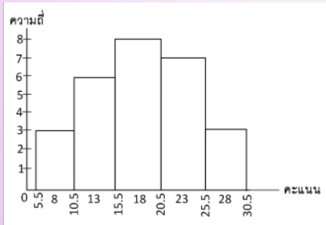
ฮิสโตแกรม (Histogram)
