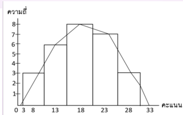
รูปหลายเหลี่ยมความถี่ (Frequency Polygon)
