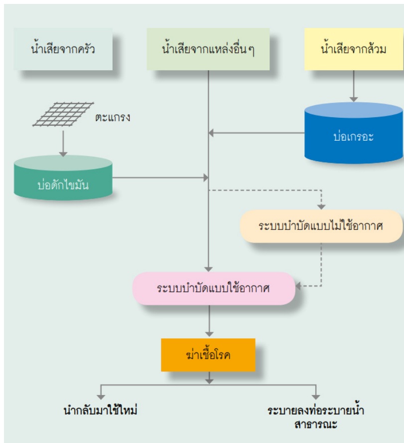
ภาพที่ 4.9 ระบบบำบัดน้ำเสียจากโรงแรม ที่มา: กรมควบคุมมลพิษ (ม.ป.ป., น. 15)
