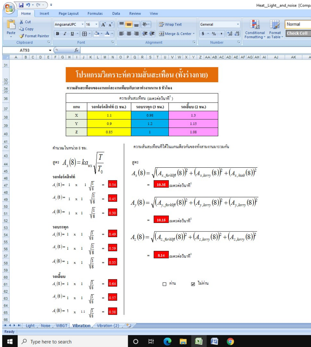
ภาพที่ 9.14 การวิเคราะห์ความสั่นสะเทือนของงานแต่ละงานเทียบกับเวลาทำงานนาน 8 ชั่วโมง
