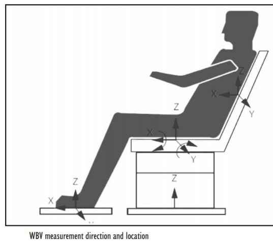
ภาพที่ 9.12 การติดตั้งวัดความสั่นสะเทือนทั้งร่างกายที่เบาะนั่งรถ ที่มา: Alphin.M.S, K.Sankaranarayanamy and S.P.Sivapirakasam, (2010)
