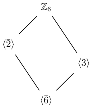
รูปที่ 2 แลตทิซของ \mathbb{Z}_6
