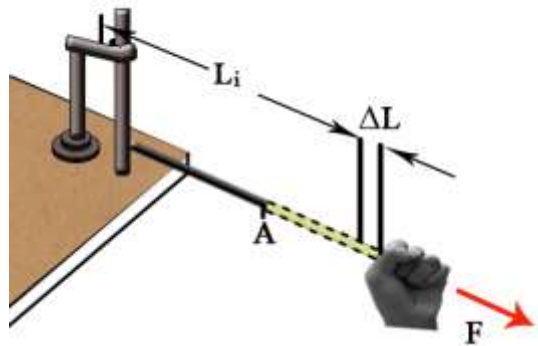
ภาพที่ 10.10 วัตถุได้รับแรงดึงจะมีความเครียดเชิงเส้น
