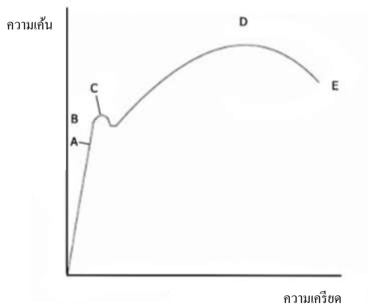
ภาพที่ 10.15 กราฟแสดงความสัมพันธ์ระหว่างความเค้นกับความเครียดของวัตถุ
