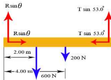
ภาพที่ 10.6 การแยกแรง
